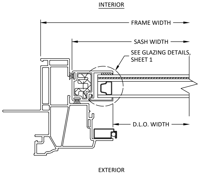
F 4 HORIZONTAL SECTION SASH JAMB
