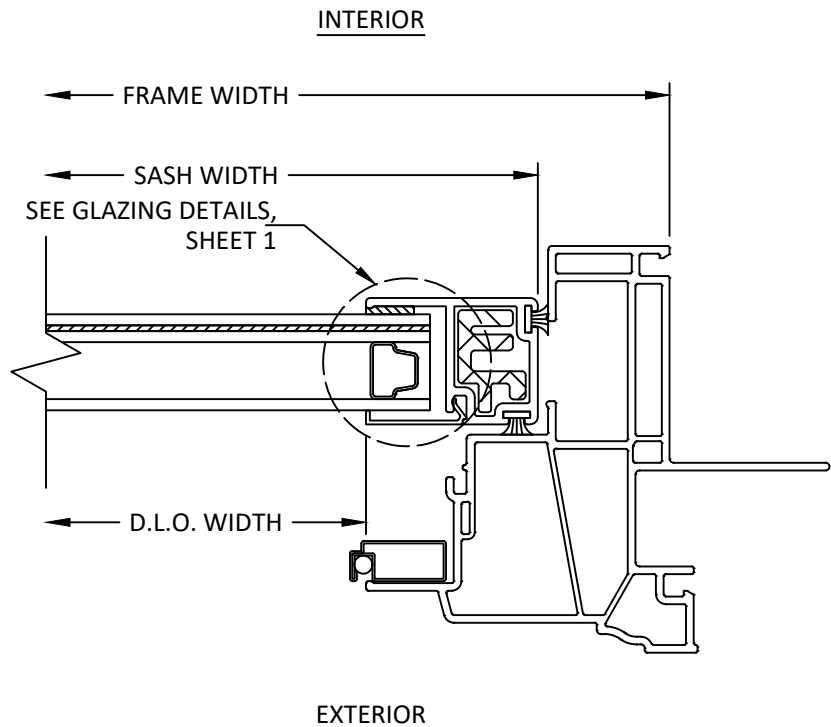
G 4 HORIZONTAL SECTION SASH JAMB
